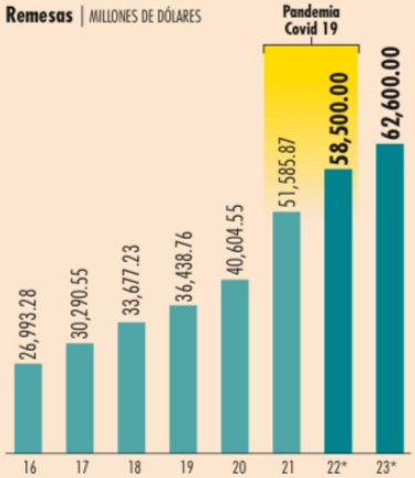
* Estimado FUENTE: BANCO DE MÉXICO GRÁFICO EE
