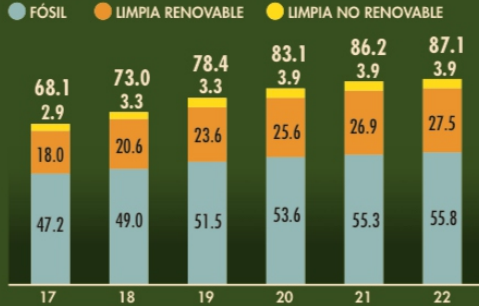
México | Capacidad de generación eléctrica | MILES DE MW
