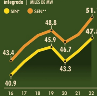
México | Demanda eléctrica máxima integrada | MILES DE MW
